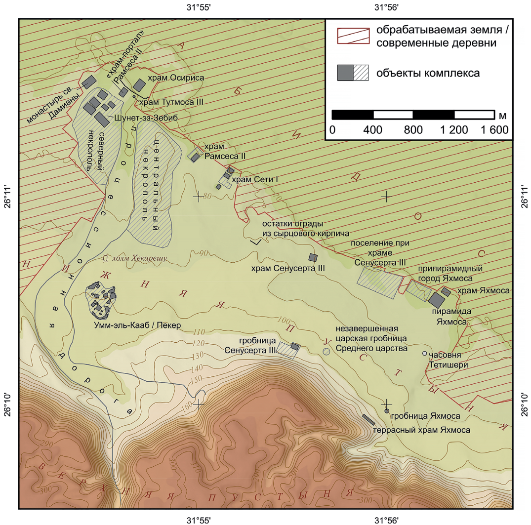
Ил. 2. Карта-схема основных археологических памятников Абидоса
