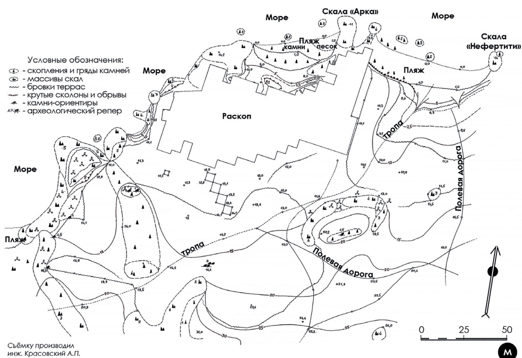
Ил. 4. Топо съемка комплекса Генеральское-Западное с границами раскопов.
