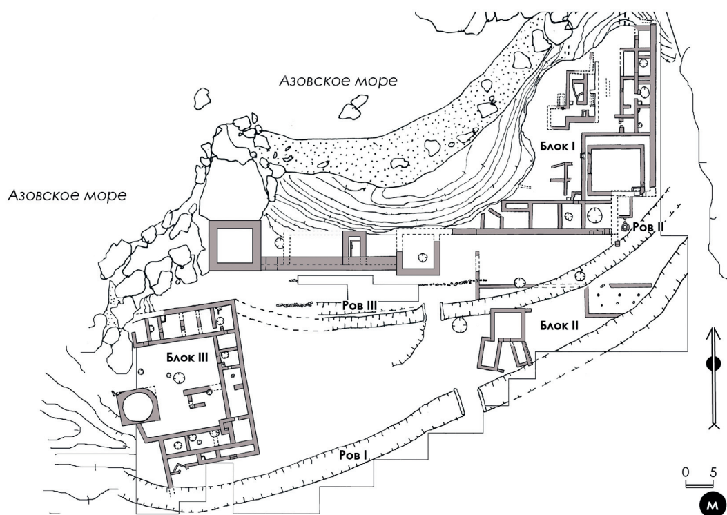
Ил. 5. План-схема строительных остатков усадебного комплекса Генеральское-Западное.
